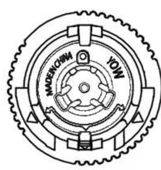
旋钮扣组件
